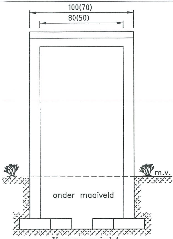
Vooraanzicht
