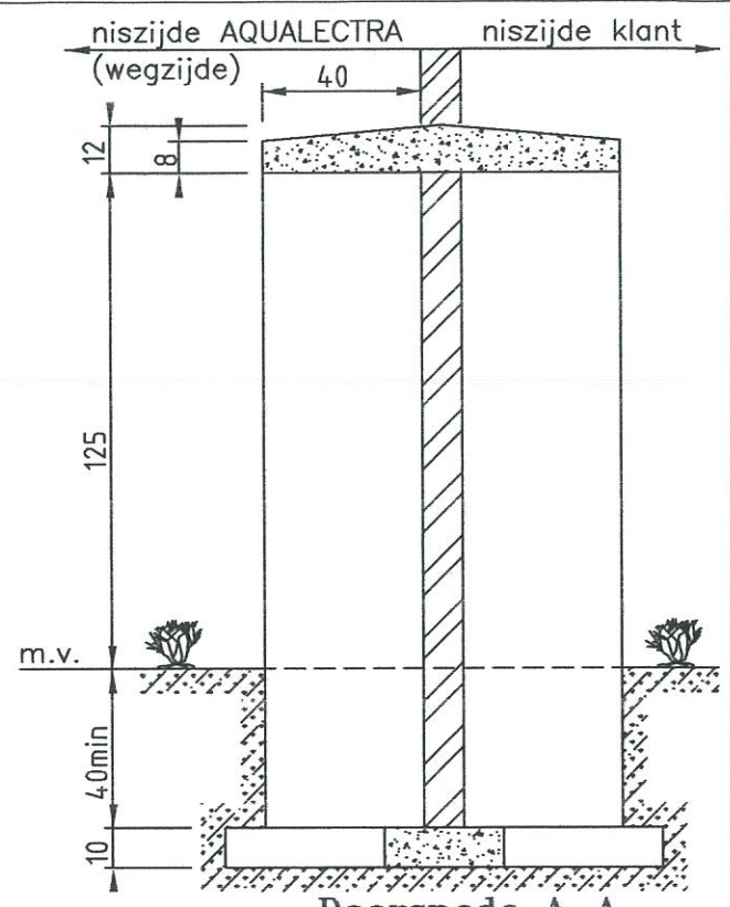
Doorsnede A-A
